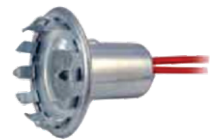
SOQUETE GARRA 2 PÓLOS, LÂMPADA 1034 FIO DE 13CM
